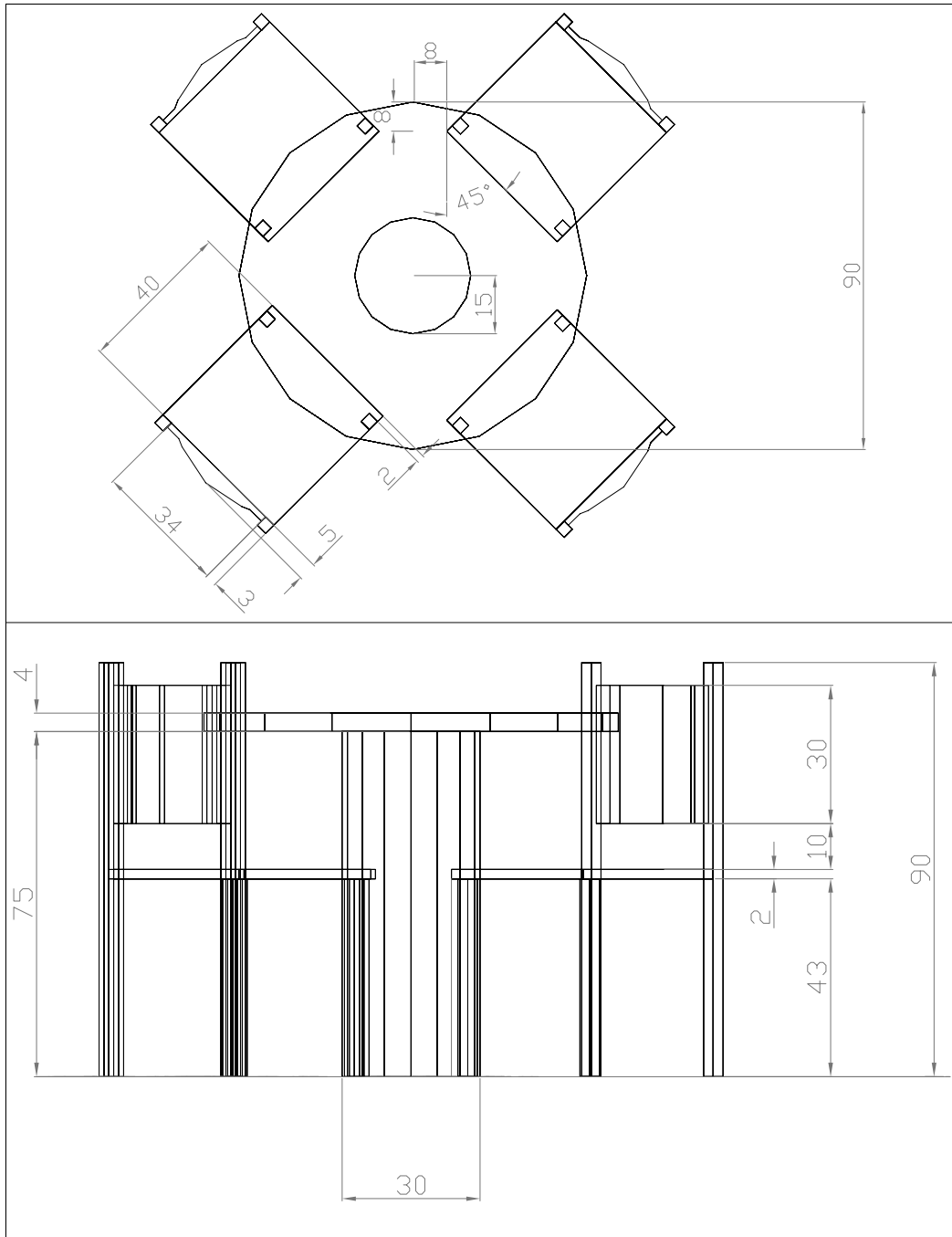
7ª PRÁCTICA DE AUTOCAD 1º BACH "A". OBJETOS TRIDIMENSIONALES: MESA Y SILLAS DE COMEDOR. S/E.
