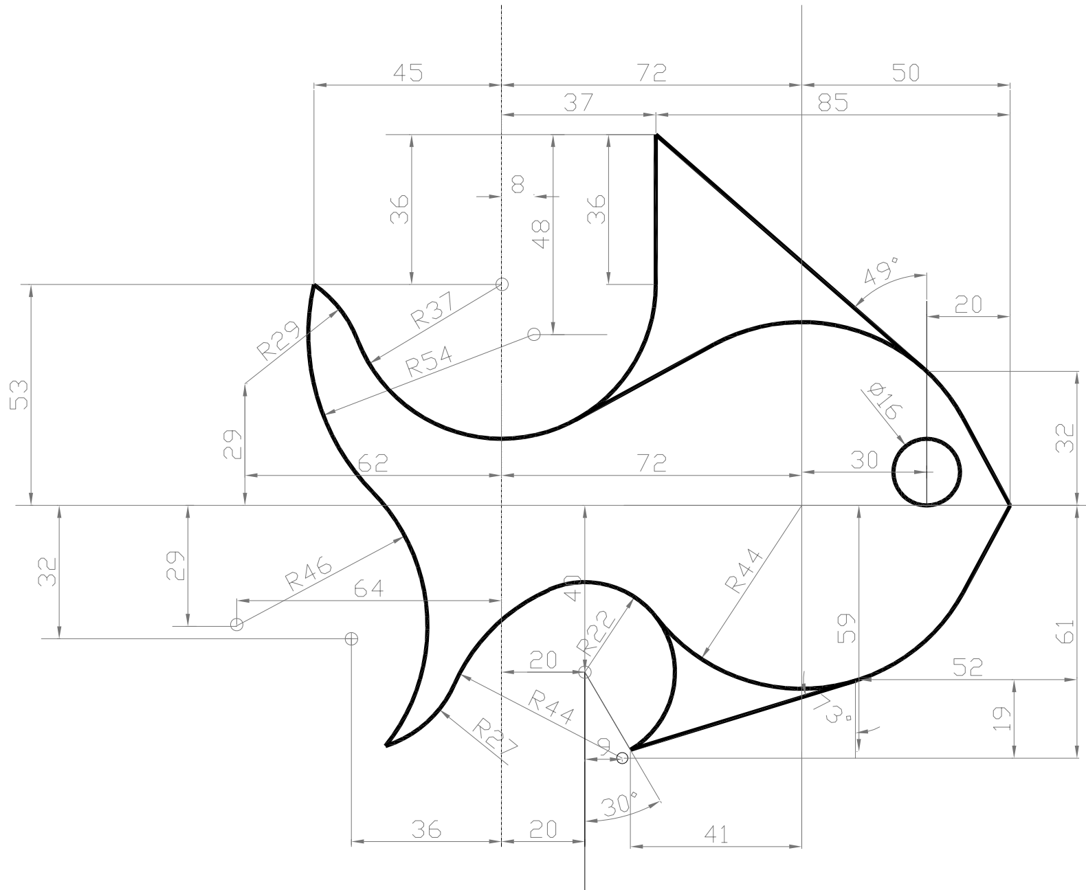
4ª PRÁCTICA DE AUTOCAD 1º BACH "A". POLILÍNEAS, CURVAS Y TANGENCIAS: PEZ. S/E.
